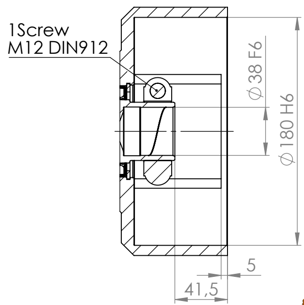
DETAIL C SECTION B-B MAßSTAB 1 : 1.5
