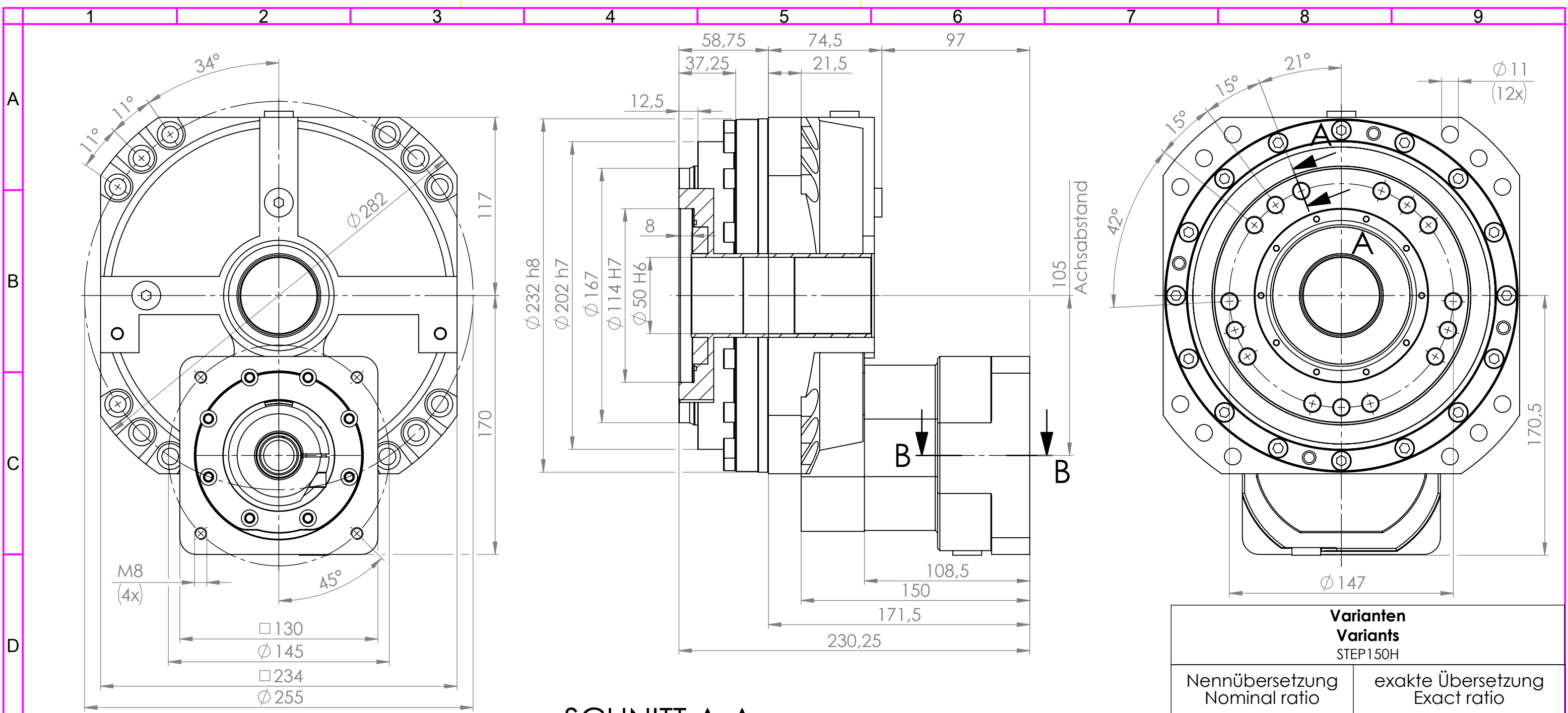
SCHNITT A-A
