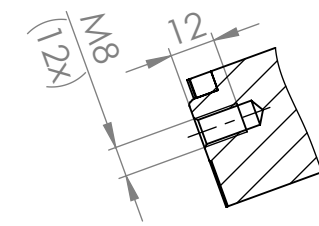
SCHNITT A-A
