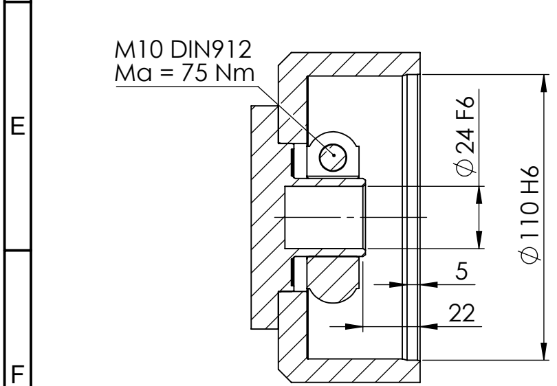
SCHNITT C-C
