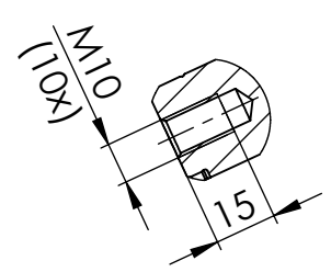
SCHNITT A-A
