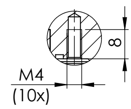
SCHNITT B-B MAßSTAB 1 : 1
