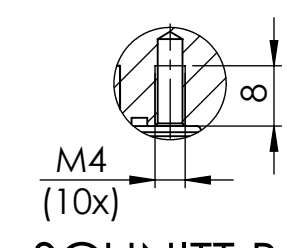
SCHNITT B-B MAßSTAB 1 : 1
