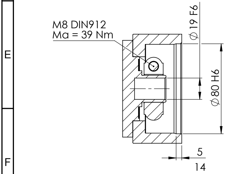
SCHNITT C-C
