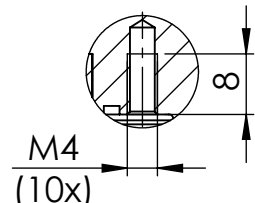
SCHNITT B-B MAßSTAB 1 : 1
