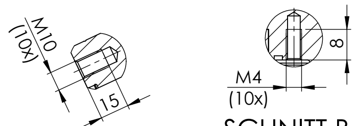
SCHNITT B-B MAßSTAB 1 : 1
