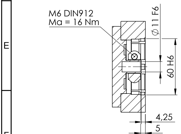
SCHNITT C-C
