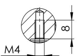
SCHNITT B-B MAßSTAB 1:1
