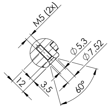
SCHNITT F-F
