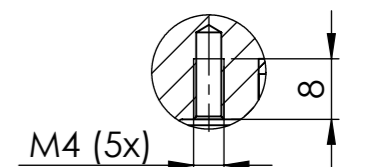
SCHNITT F-F MAßSTAB 1 : 1
