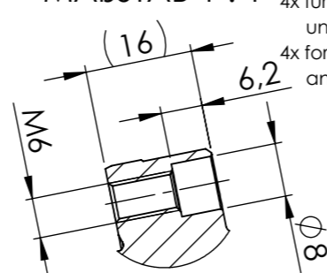
SCHNITT E-E MAßSTAB 1 : 1
