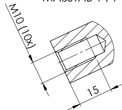
SCHNITT E-E MAßSTAB 1 : 1
