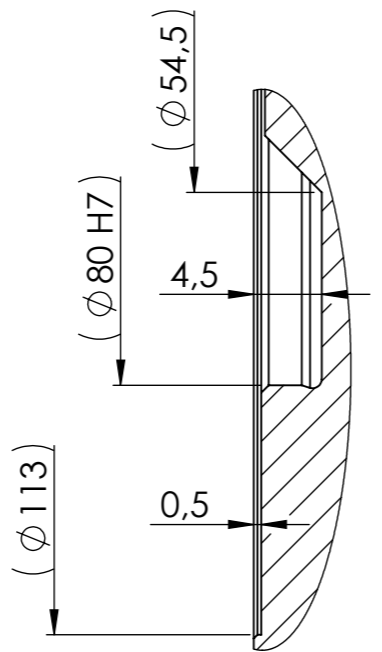
DETAIL A MAßSTAB 2 : 1
