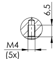
SCHNITT B-B MAßSTAB 1 : 1
