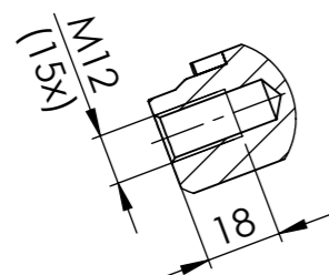
SCHNITT A-A MAßSTAB 1 : 2
