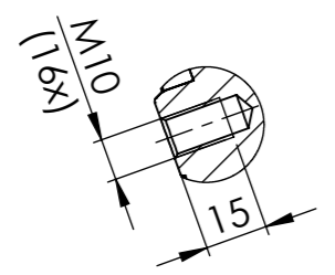
SCHNITT B-B MAßSTAB 1 : 2
