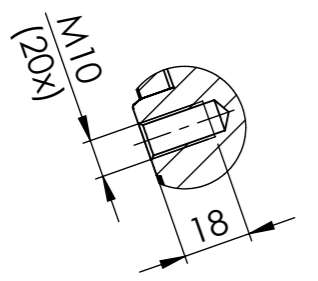
SCHNITT B-B MAßSTAB 1 : 2
