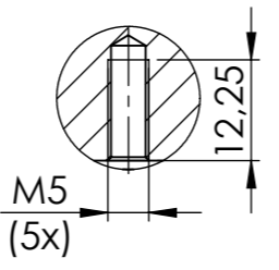
SCHNITT B-B MAßSTAB 1 : 1
