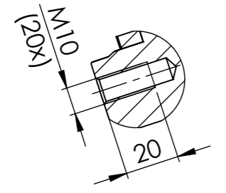
SCHNITT A-A MAßSTAB 1 : 2
