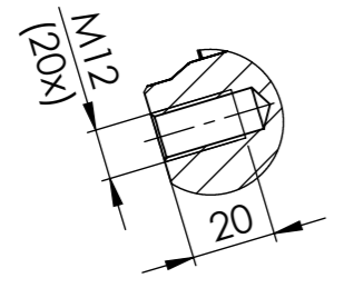
SCHNITT A-A MAßSTAB 1:2
