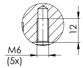
SCHNITT B-B MAßSTAB 1:1
