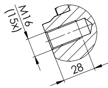
SCHNITT A-A MAßSTAB 1 : 2
