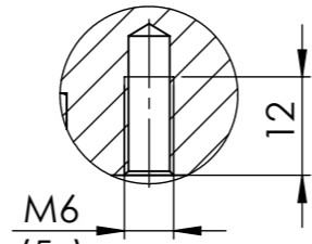
SCHNITT B-B MAßSTAB 1 : 1
