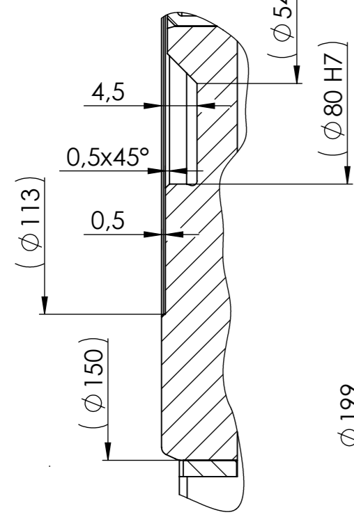
DETAIL D MABSTAB 1.5 : 1
