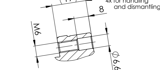
SCHNITT E-E MABSTAB 1 : 1
