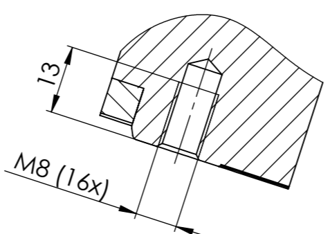
SCHNITT E-E MABSTAB 1 : 1
