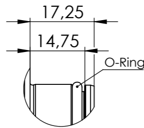
DETAIL B MAßSTAB 1 : 1
