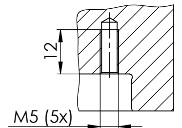
SCHNITT F-F MAßSTAB 1 : 1
