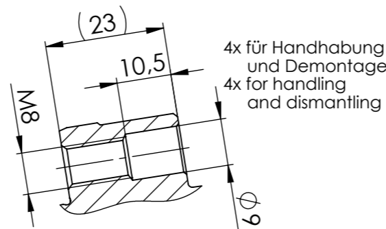
SCHNITT E-E MAßSTAB 1 : 1
