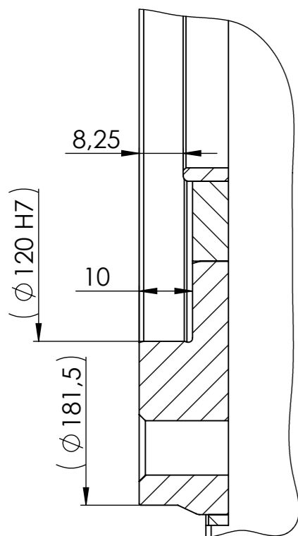
DETAIL D MAßSTAB 1 : 1
