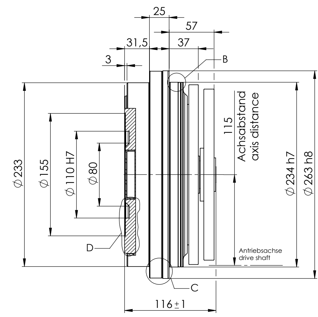
SCHNITT A-A MAßSTAB 1 : 1
