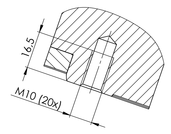
SCHNITT E-E MAßSTAB 1 : 1
