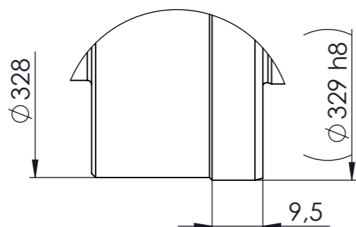
DETAIL C MAßSTAB 1 : 1
