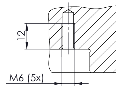
SCHNITT F-F MAßSTAB 1 : 1
