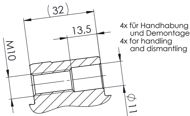
SCHNITT E-E MAßSTAB 1 : 1
