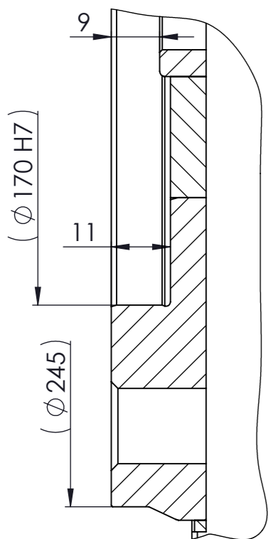
DETAIL D MAßSTAB 1 : 1
