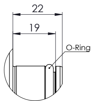
DETAIL B MAßSTAB 1 : 1
