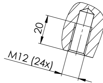
SCHNITT A-A MABSTAB 1 : 1.5
