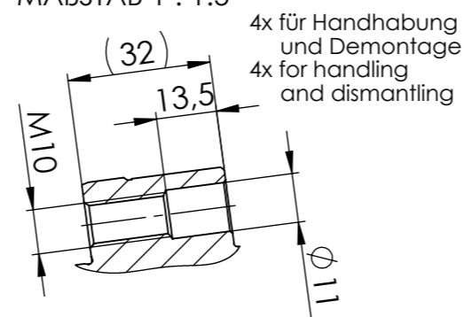
SCHNITT E-E MABSTAB 1 : 1.5
